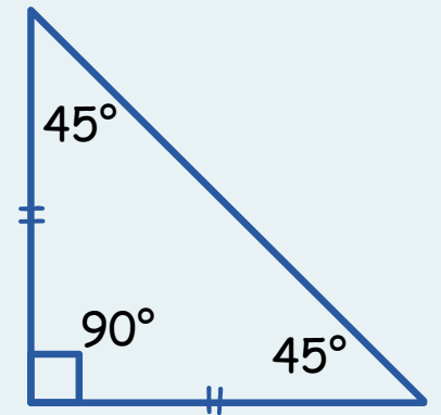
Triangle rectangle isocèle
