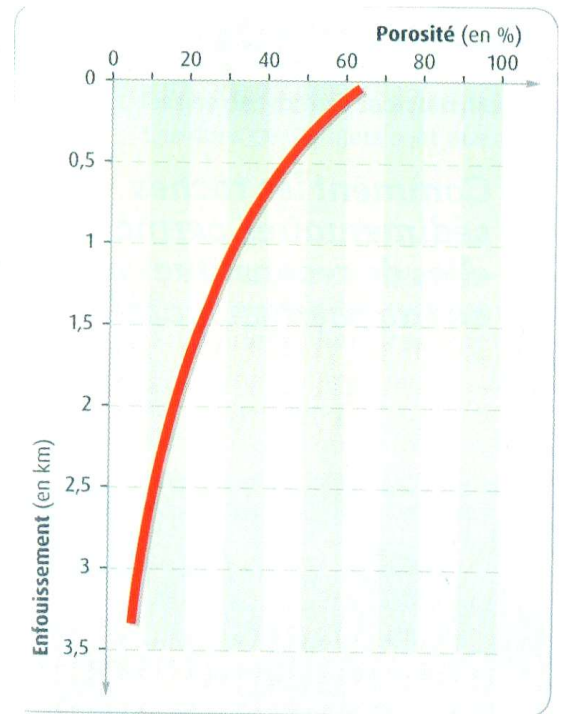
Document 7b : Evolution de la porosité des sédiments en fonction de la profondeur
