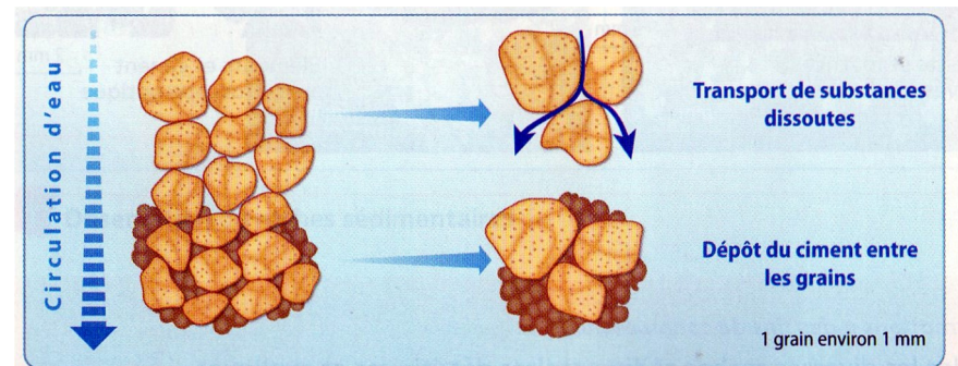
Document 7a : La diagenèse : transformation des sédiments en roche sédimentaire (compaction et cimentation)
