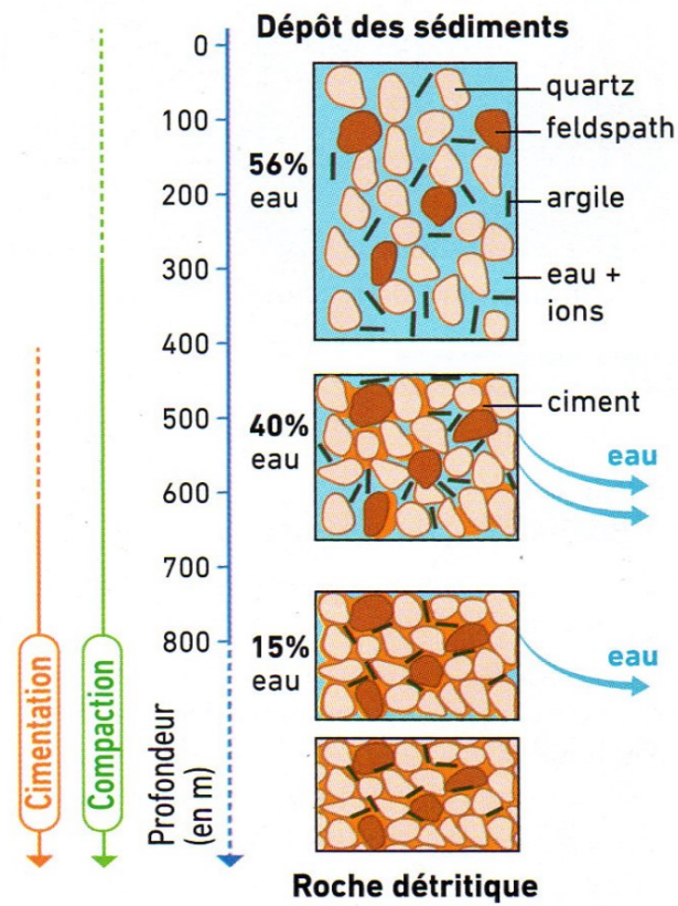
Document 7a : La diagenèse : transformation des sédiments en roche sédimentaire (compaction et cimentation)
