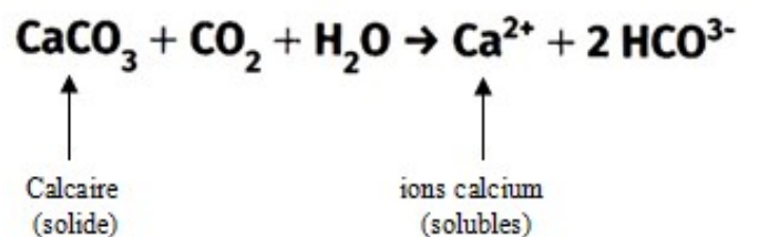
Document 3 : réaction de dissolution du calcaire
