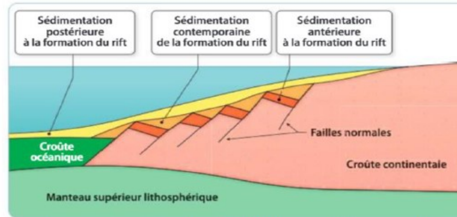
Marge passive (blocs basculés délimités par failles normales)
