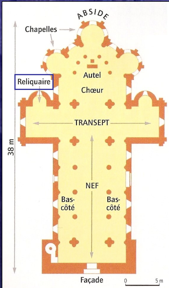
Plan de l'église romane de Saint-Nectaire
