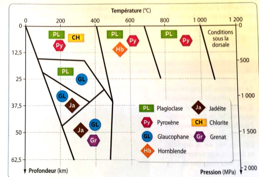
3 Diagramme pression-température de stabilité des minéraux des (méta)gabbros
