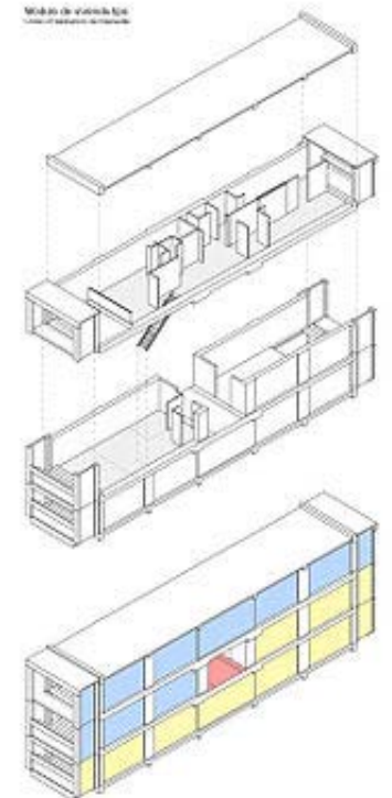
Module de logement de l'unité d'habitation de Marseille connue sous le nom de Cité radieuse, 1947-1952
