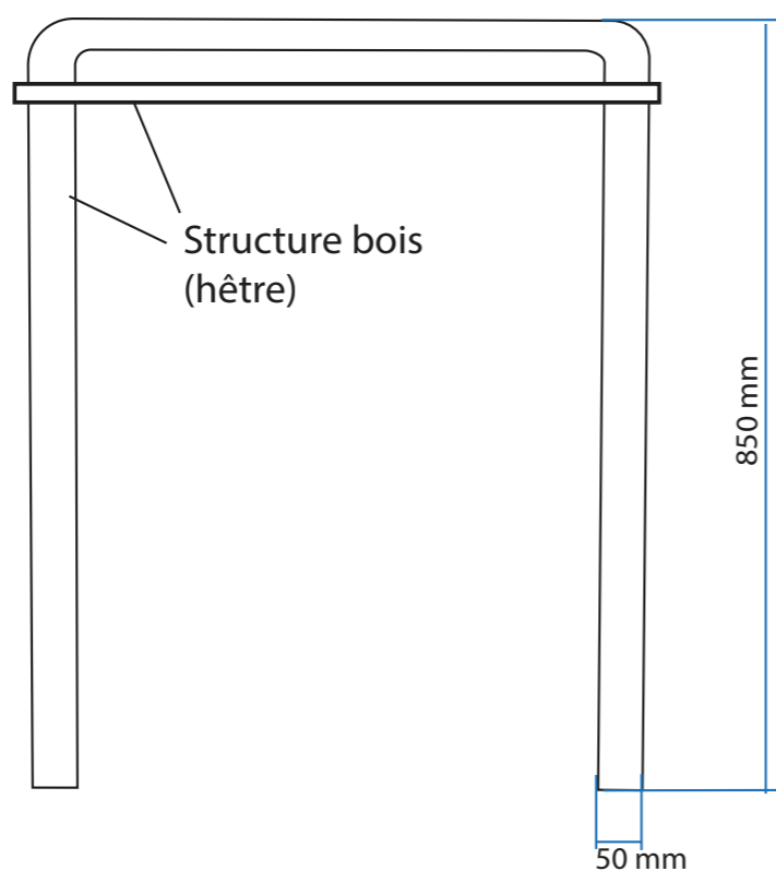
Vue arrière
