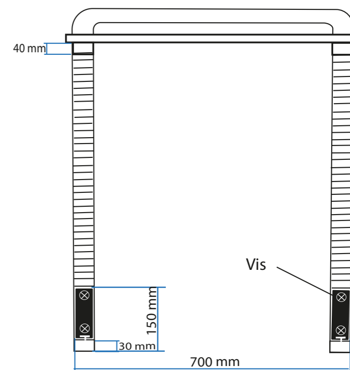
Vue face
