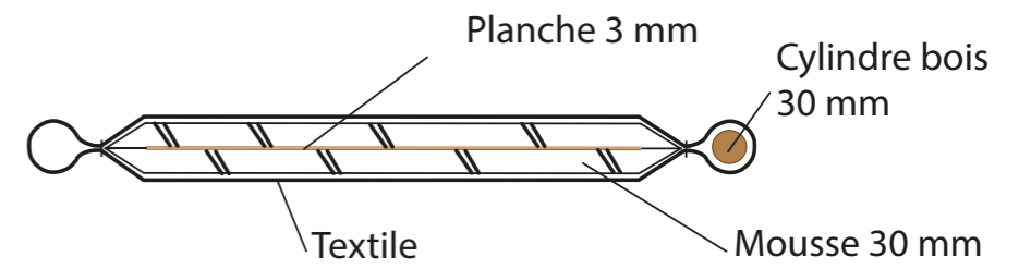
Vue de coupe A-A
