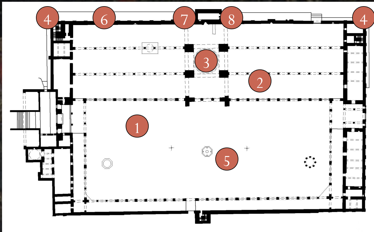
Le plan de la mosquée de Damas
