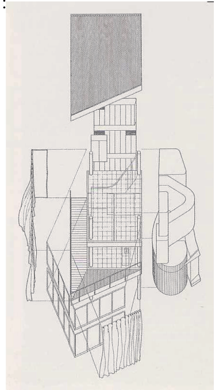
Maison poteau
