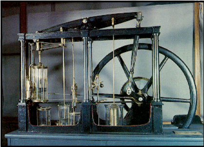
↑ Machine à vapeur de Watt, deuxième moitié du XVIIIème s.
