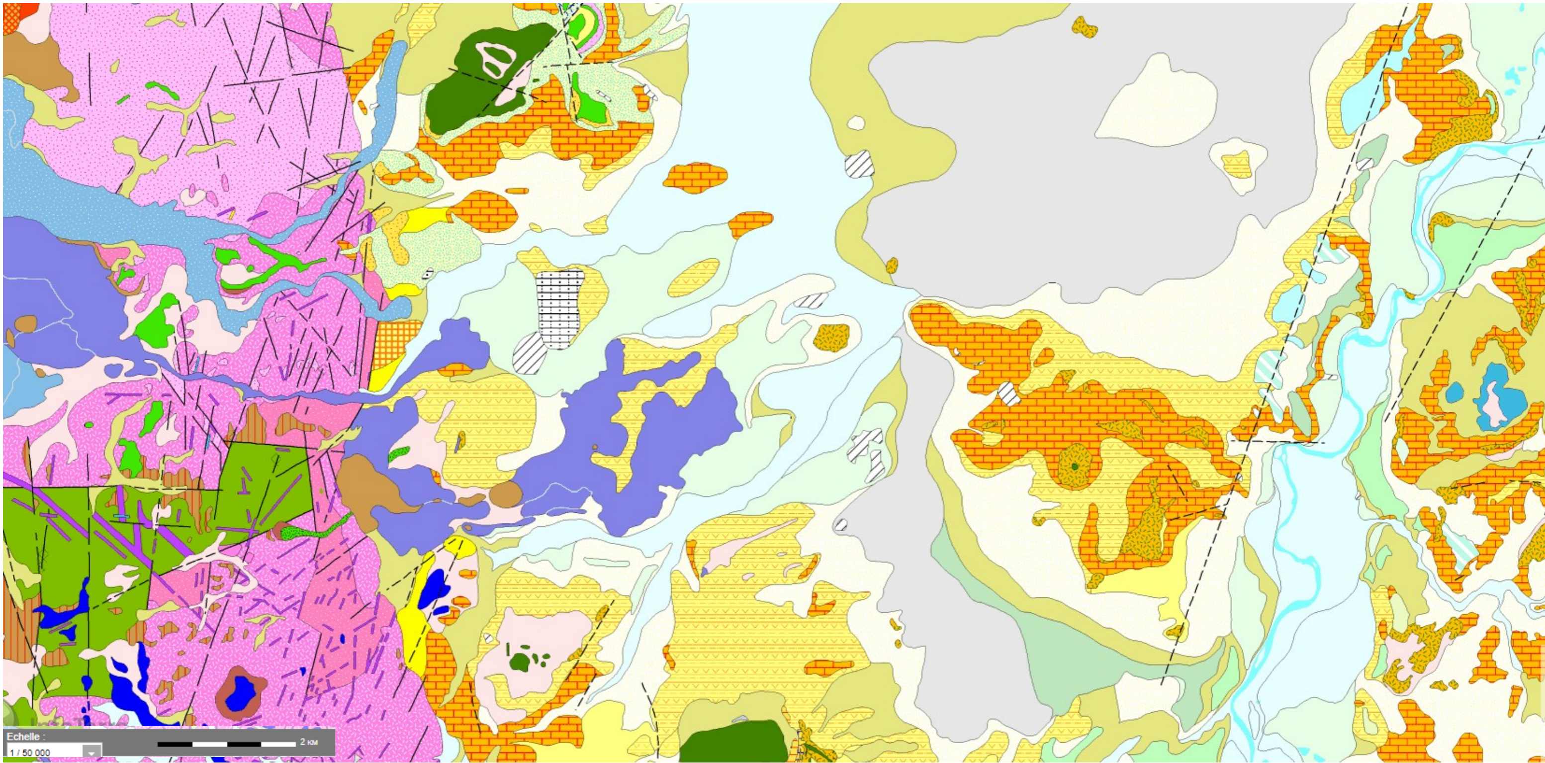
Carte géologique simplifiée de la région de Clermont Ferrand (issue des carte du BRGM )
