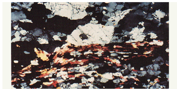
Lame mince de migmatites (roches de la zone F6). Zone grise = leucosome (gros minéraux de quartz et feldspath cristallisés après fusion). Zone colorée = mélanosome (petits minéraux de biotite et sillimanite qui n'ont pas fondu).
