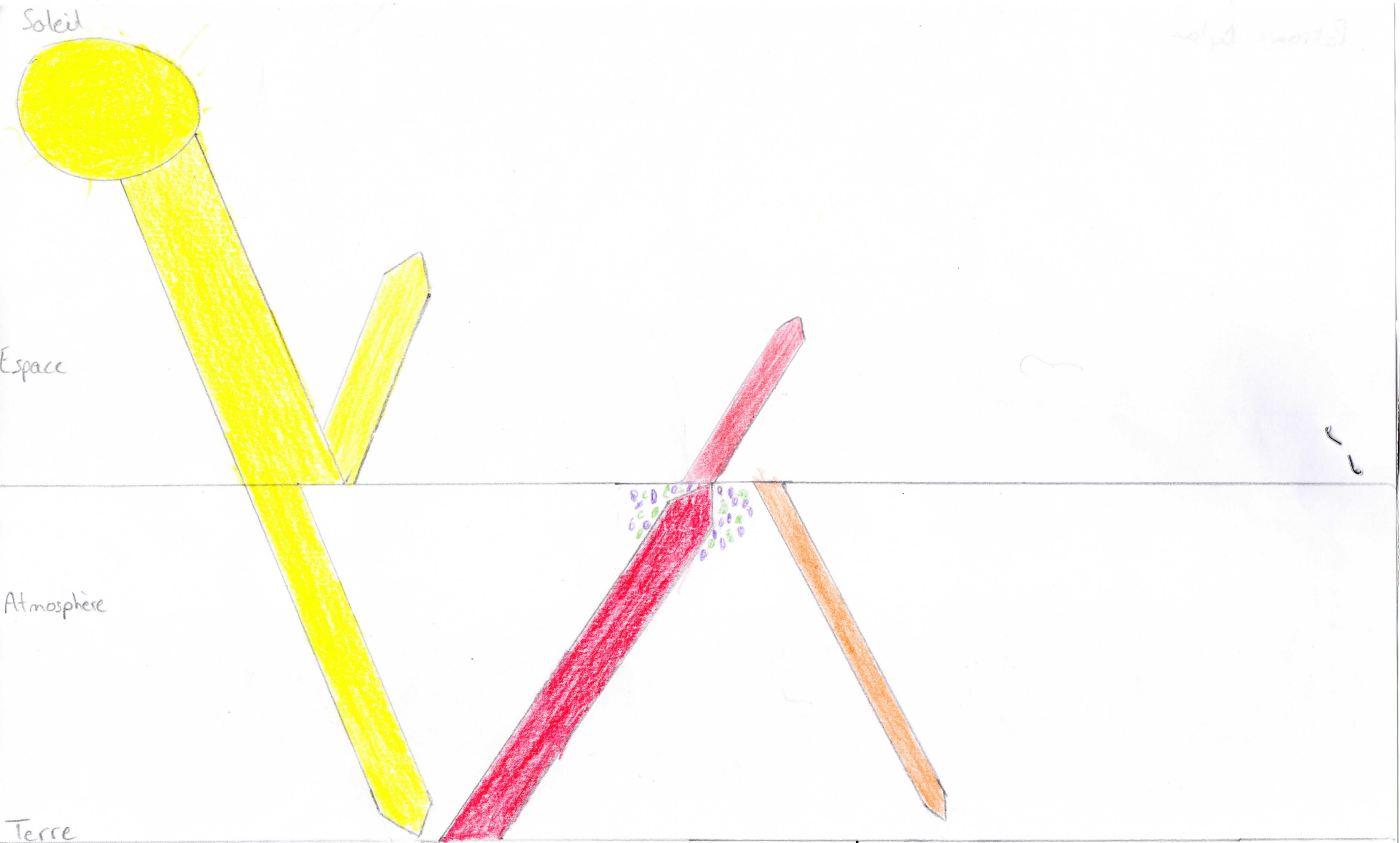
Titre : Schéma représentant l'effet de serre sur la Terre.
