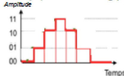
Exemple : signal numérique codé sur 2 bits ; Il ne peut avoir que 4 valeurs codées en binaire au cours du temps, 00,01,10,11
